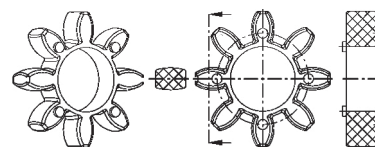
XL4 型以下梅花形弹性体轴向直齿面，中间有腹板
