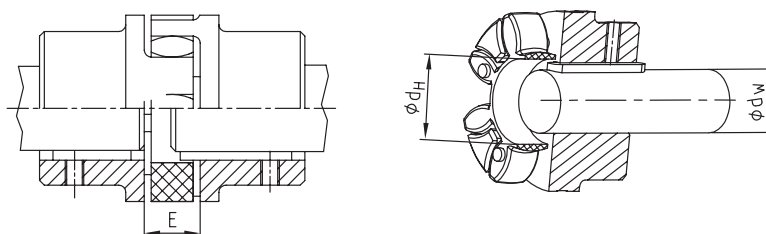
安装尺寸
