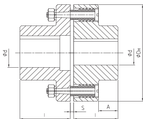
TL 弹性套柱销式联轴器的基本选型参数和主要尺寸
