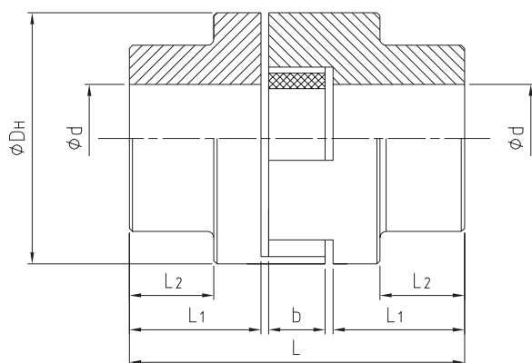
ML 梅花弹性联轴器的基本选型参数和主要尺寸
