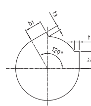
D 圆柱型孔普通 切向键键槽
