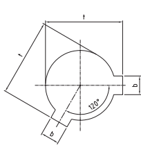
B 型 120 度布置平键 双键槽
