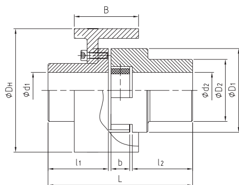
MLL 制动轮式梅花弹性联轴器的基本选型参数和主要尺寸
