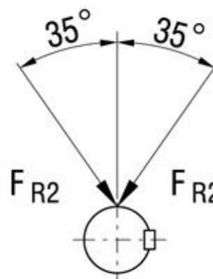
允许的作用力方向 Permissible direction of force
