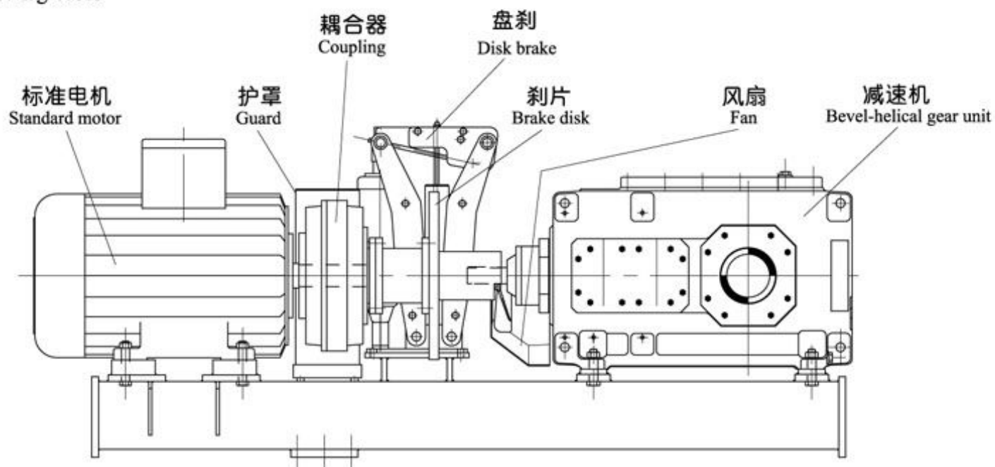
带齿轮箱摆动底座 Gear unit swing-bases
