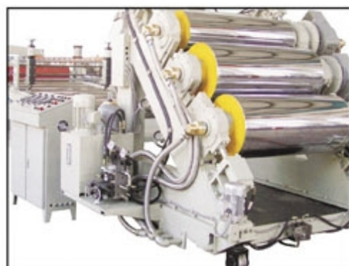
三辊压光机
